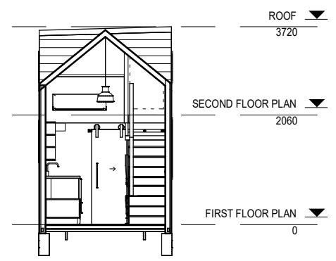
3 SECTION 02 03 1 : 100
