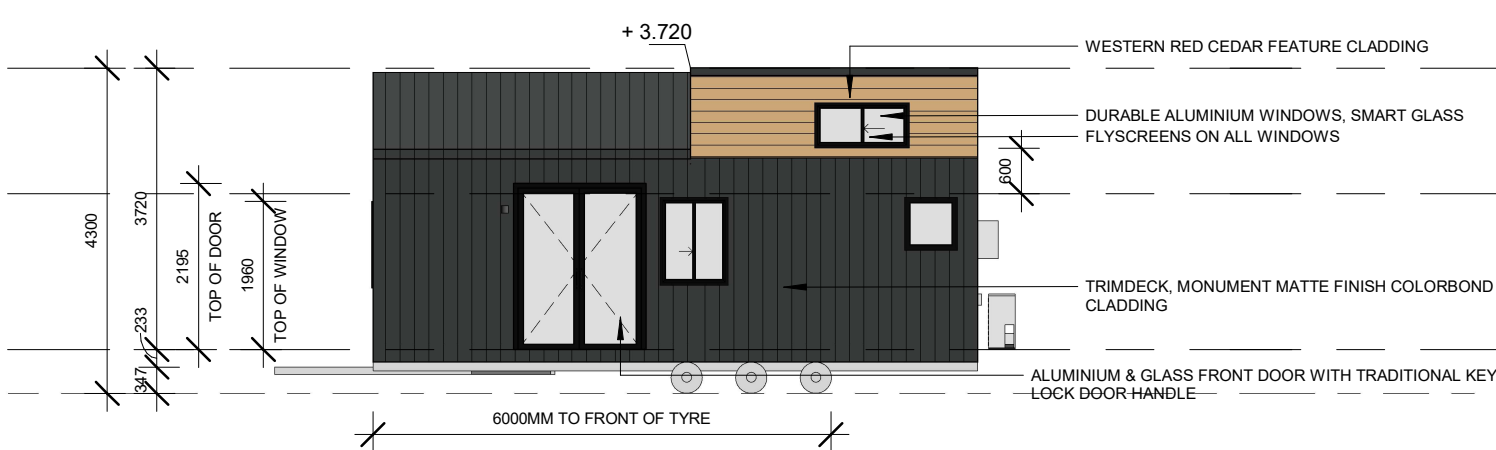
3 ELEVATION 03 03 1 : 100
