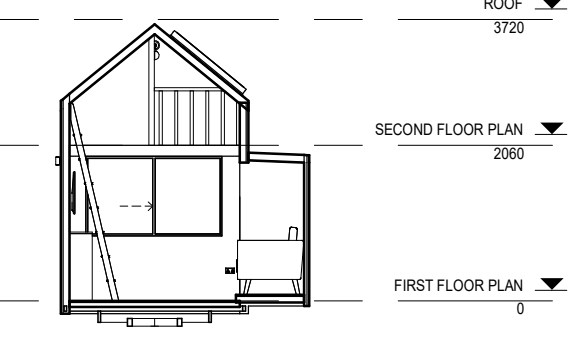
4 SECTION 04 03 1 : 100
