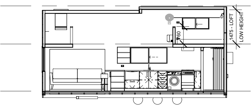
2 SECTION 03 03 1 : 100
