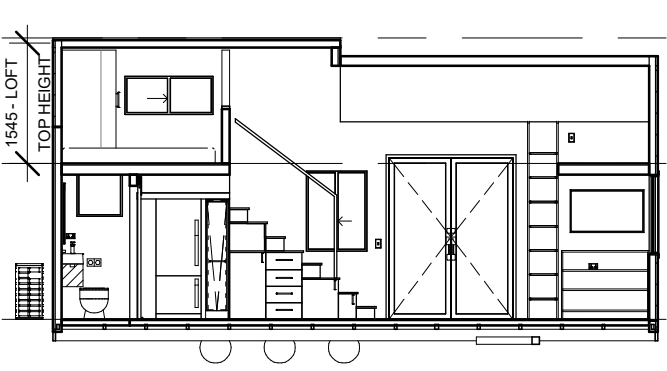
1 SECTION 01 03 1 : 100
